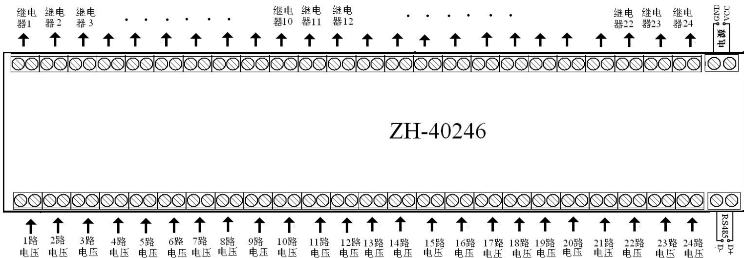
图四、产品接线参考图
