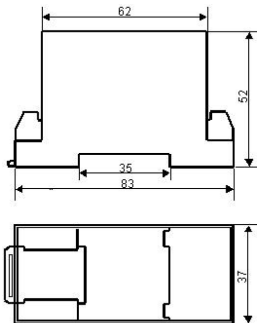
图 4.2、产品尺寸图
